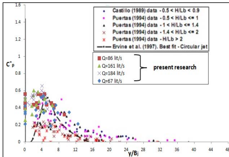
شکل ۹- ضریب مقادیر حدی منفی C_p^- در مقابل \frac{Y}{B_j}
