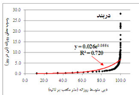
شکل ۲- منحنی سنج رسوب داده‌های اولیه در ایستگاه‌های هیدرومتری مورد مطالعه
