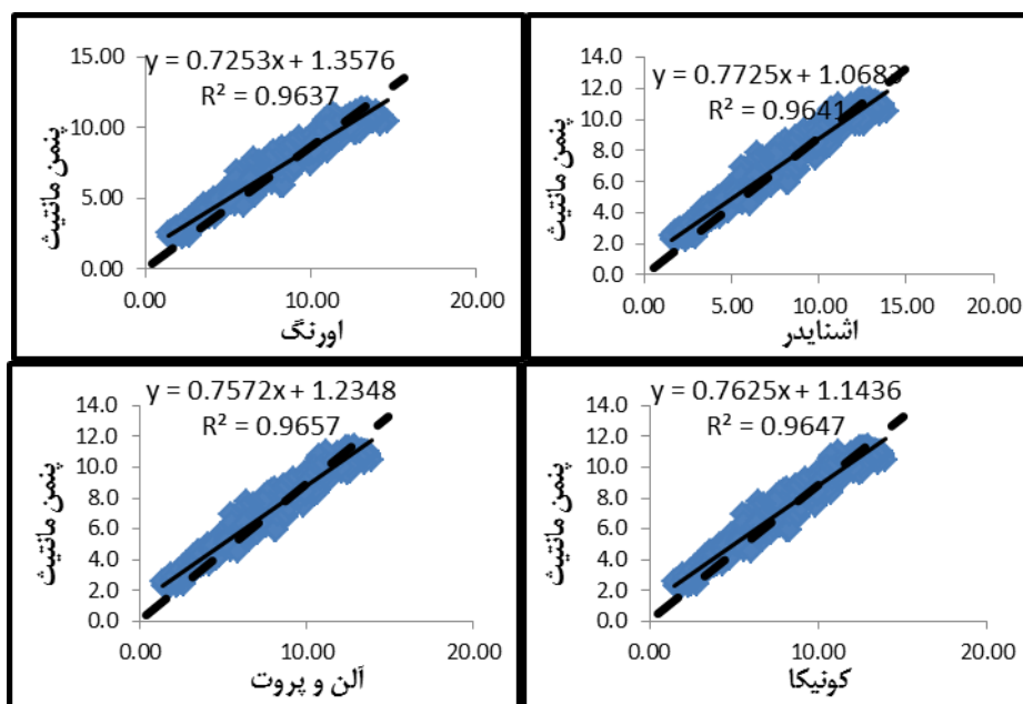
شکل ۲- نمودار همبستگی بین مقادیر تبخیر و تعرق پتانسیل (میلی متر بر روز) برآورد شده از روش پهنم مانتیث و روش های اورنگ (۱۹۹۸)، اشنایدر (۱۹۹۲)، کونیکا (۱۹۸۹) و آلن و پروت (۱۹۹۱) به صورت روزانه، در سال های ۹۱-۱۳۷۷ در ایستگاه اهواز (خط نقطه چین خط یک به یک و خط دیگر بهترین خط برازش شده).
