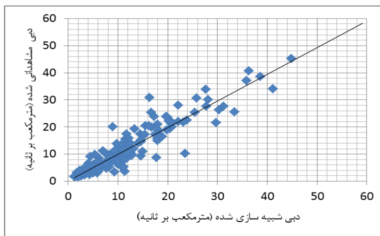
شکل ۳- پراکنش داده های واقعی و شبیه سازی شده در دوره آموزش
