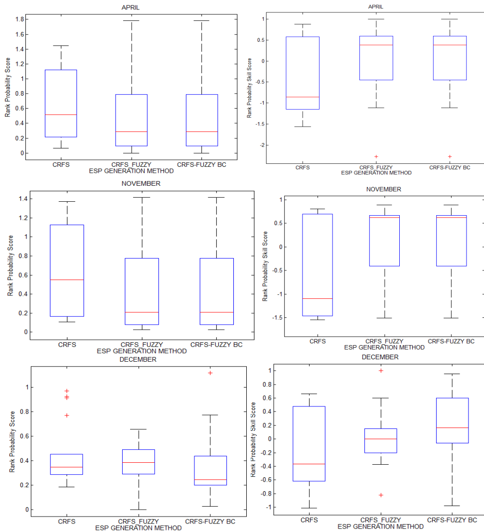
شکل ۵- نمودار تغییرات امتیاز احتمالاتی رتبه ای و امتیاز مهارت برای ماههای پیش‌بینی در طول دوره ارزیابی ۸۰-۱۳۵۳
