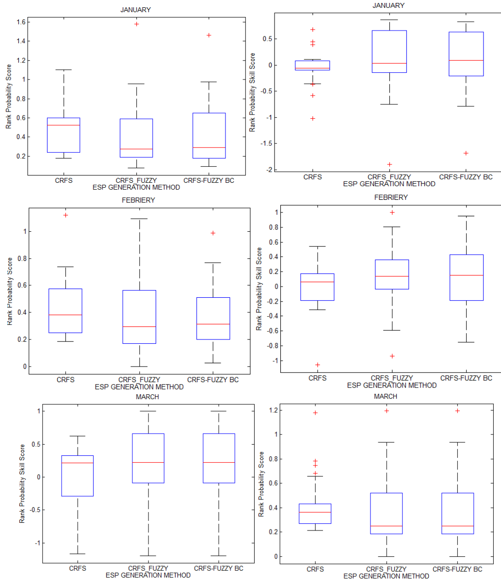
ادامه شکل ۵- نمودار تغییرات امتیاز احتمالاتی رتبه ای و امتیاز مهارت برای ماه‌های
