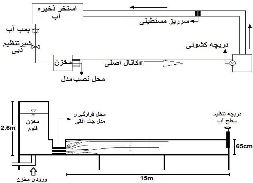
شکل ۱- پلان و مقطع طولی فلوم آزمایشگاهی مورد استفاده در این مطالعه
