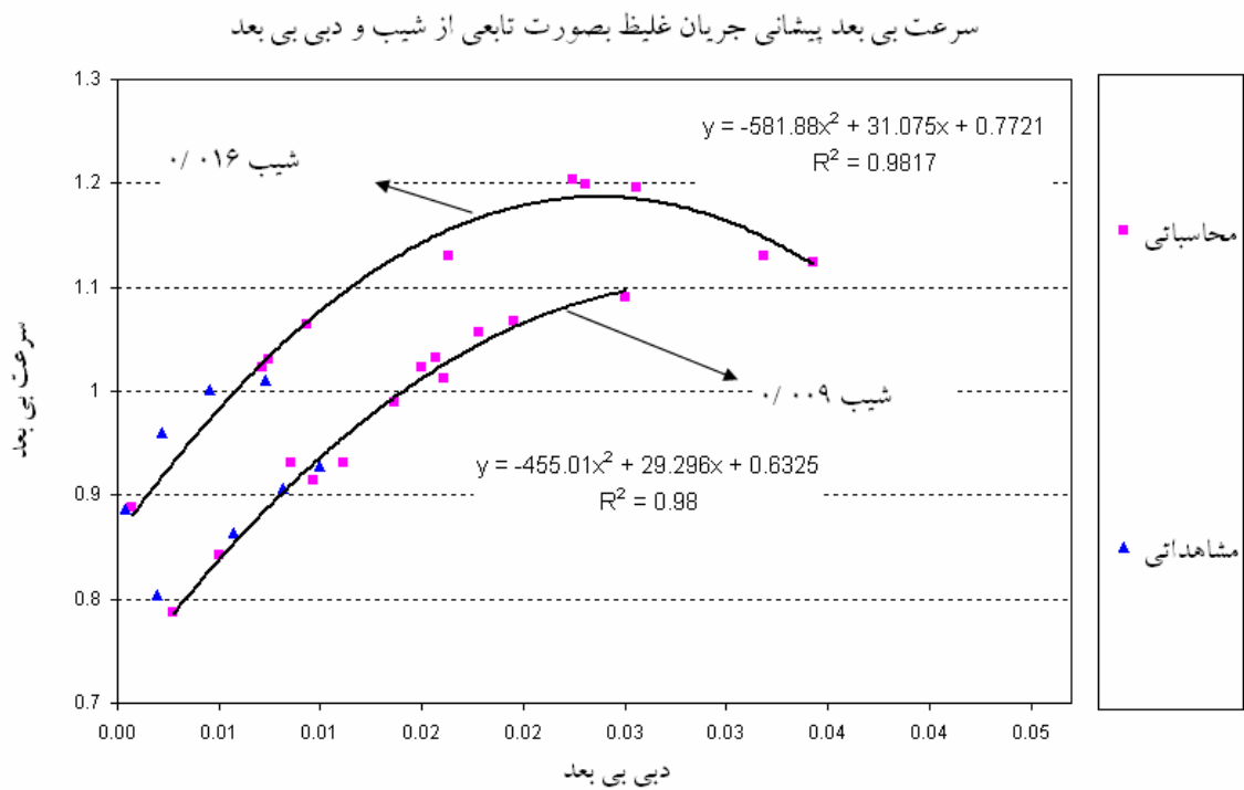
شکل شماره 12- رابطه با دبی بی بعد با سرعت بی بعد پیشانی جریان غلیظ در واگرایی 8 درجه و در شیبهای 0/016 و 0/009
