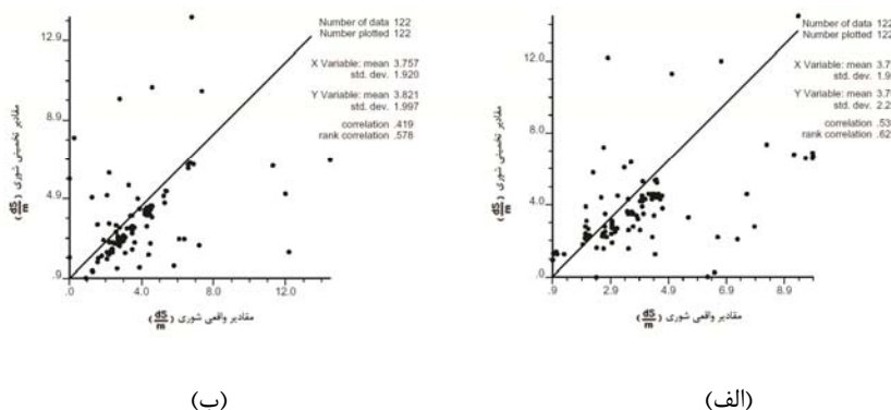
شکل ۷- نقشه پراکندگی بین مقادیر تخمین زده شده و مقادیر واقعی (الف) روش کریجینگ معمولی (ب) روش کریجینگ شاخص
