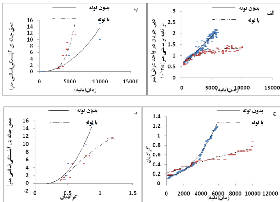
شکل ۱۳- دانه‌بندی ۲-۱ میلی‌متر در دو حالت با و بدون لوله، الف: دبی جریان در واحد عرض در طول زمان، ب: عمق چاله‌ی آبستگي در طول زمان، ج: گراديان در مقابل زمان، د: عمق چاله‌ی آبستگي در مقابل گراديان.
