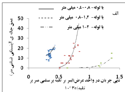
شکل ۱۰- نمودار عمق چاله‌ی آبخستگی در مقابل گرادیان و دبی جریان برای هر سه دانه بندی در حالت با لوله، الف: عمق چاله آبخستگی در مقابل دبی جریان در واحد عرض، ب: عمق چاله آبخستگی در مقابل گرادیان.
