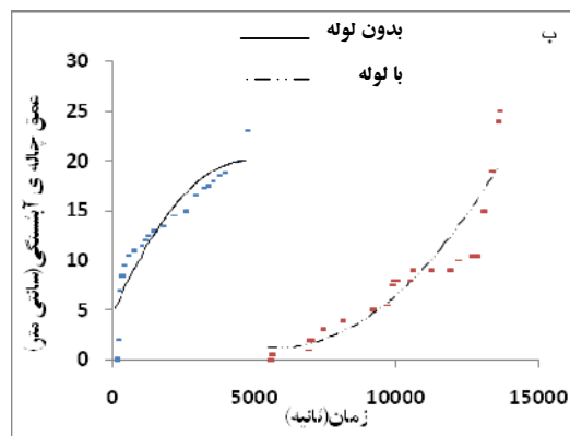
شکل ۱۱- نمودارهای مربوط به دانه بندی ۰/۸-۰/۴ میلی‌متر در دو حالت با و بدون لوله، الف: دبی جریان در واحد عرض در طول زمان، ب: عمق چاله آبستگي در طول زمان، ج: گرادیان در طول زمان، د: عمق چاله آبستگي در مقابل گرادیان
