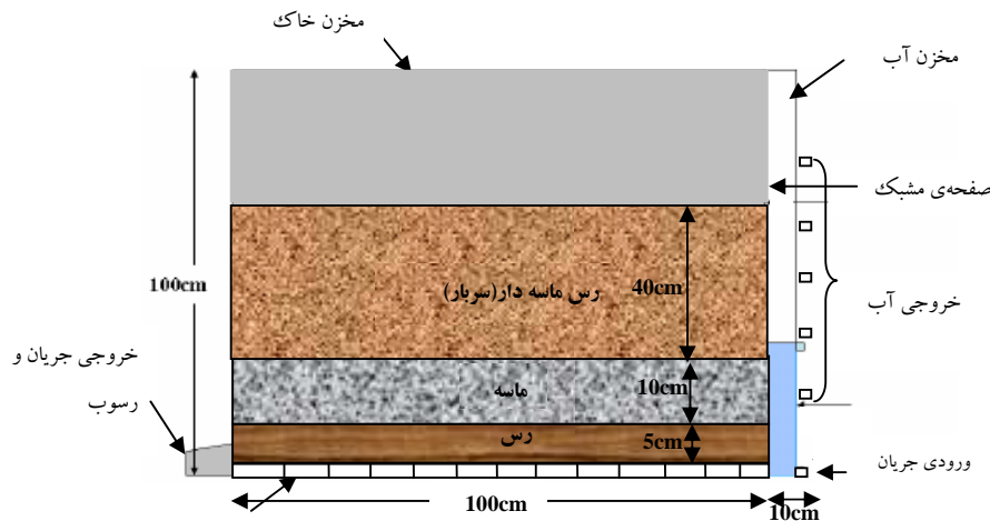
شکل ۳- نمای دستگاه
