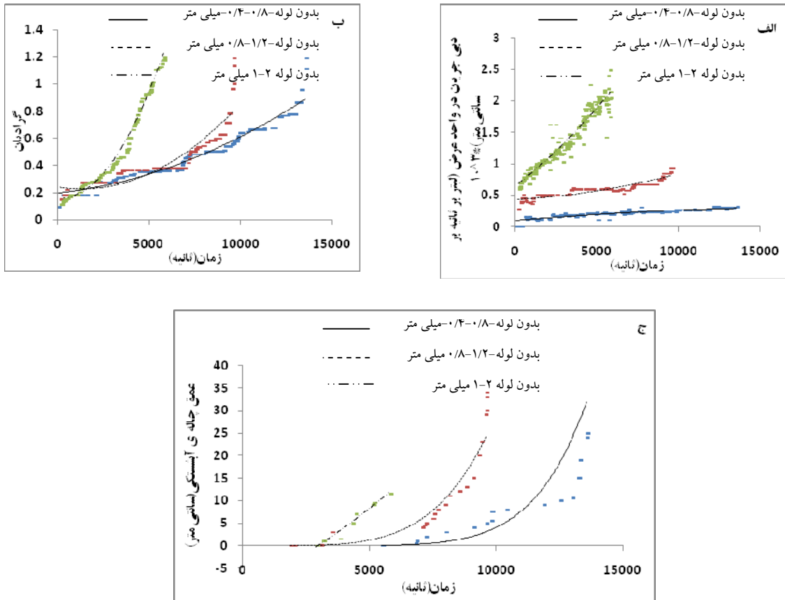
شکل ۷- نمودارهای دبی و گرادیان و عمق چاهلی آبهستگی در طول زمان برای هر سه دانه‌بندی در حالت بدون لوله، الف: دبی در طول زمان، ب: گرادیان در طول زمان، ج: عمق چاهلی آبهستگی در مقابل زمان
