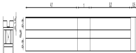
شکل ۳- پلان و مقطع کانال مرکب آزمایشگاهی
