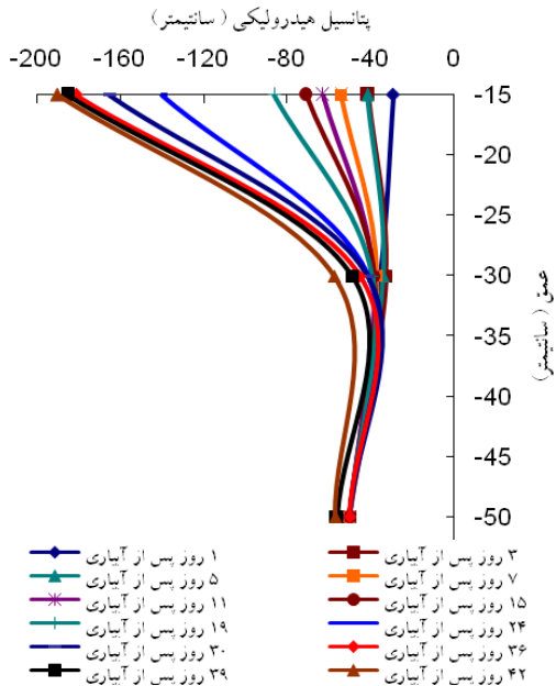
شکل ۱۳- منحنی پتانسیل هیدرولیکی- عمق درمالج سنگی ۲/۵ سانتی‌متر
