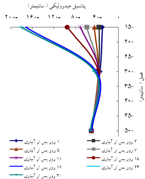
شکل ۱۱- منحنی پتانسیل هیدرولیکی- عمق در مالج لاستیکی ۲/۵ سانتی‌متر
