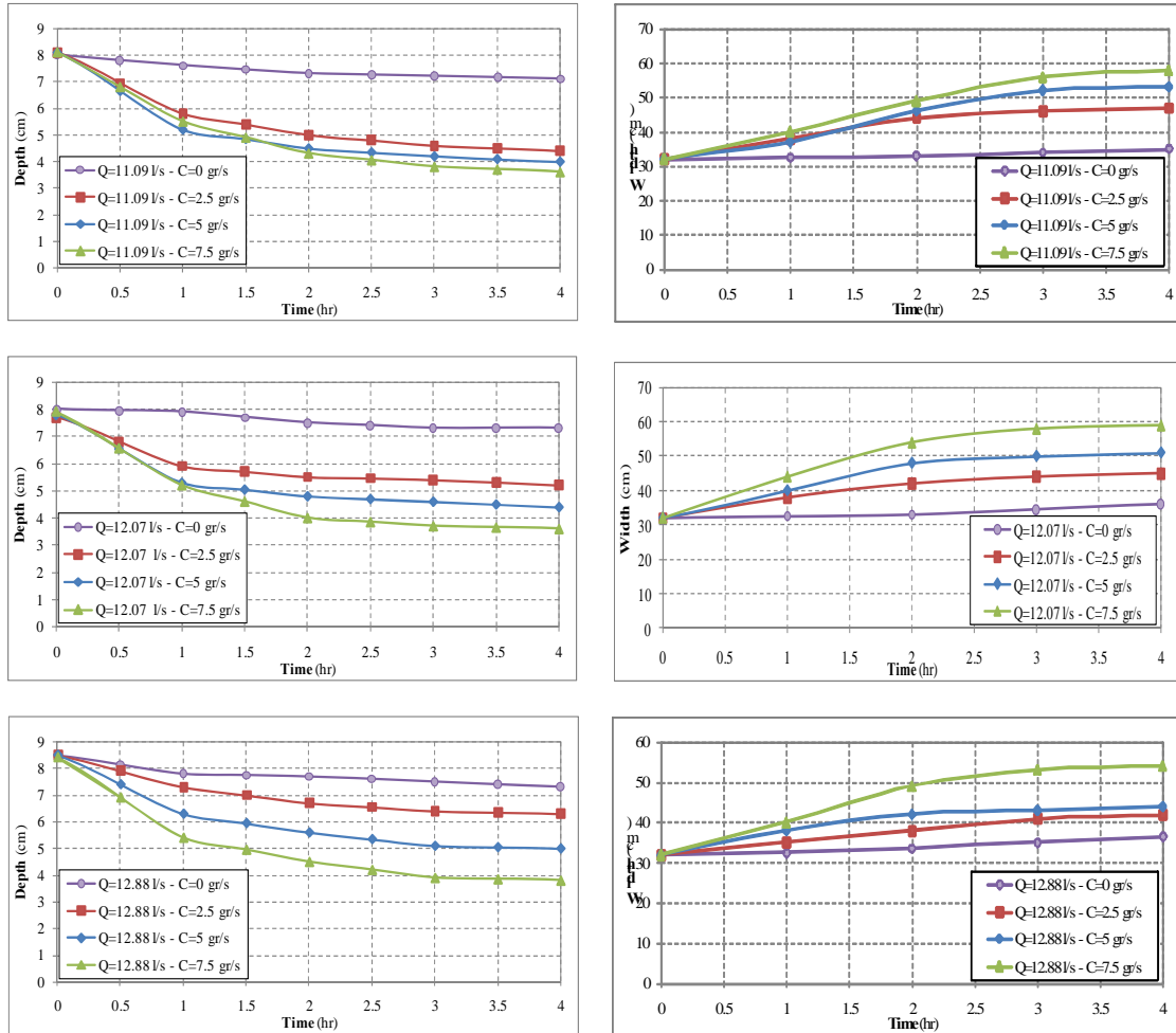
شکل ۵- نرخ تعادل عرض و عمق آبراهه در مقطع A در حالت دانه بندی با قطر متوسط ۱/۲ میلی متر
