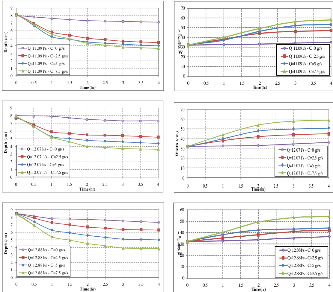
شکل ۶- نرخ تعادل عرض و عمق آبراهه در مقطع A در حالت دانه بندی با قطر متوسط ۱/۶ میلی‌متر
