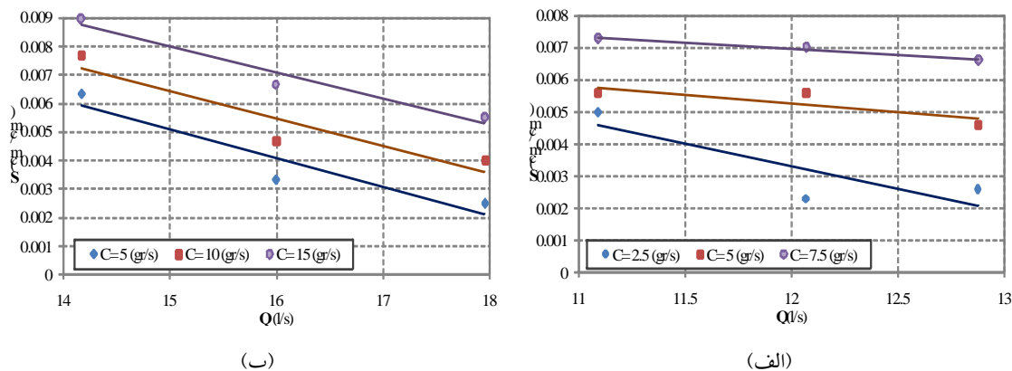
شکل ۷- تغییرات شیب کانال پایدار نسبت به تغییرات دبی جریان و رسوب، (الف) D_{50}=1/2 mm، (ب) D_{50}=1/6 mm
