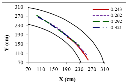
شکل ۱۱- پلان خط القعر کانال فرسایشی در قوس ۹۰ درجه برای سرریزها به ازای اعداد فرود مختلف
