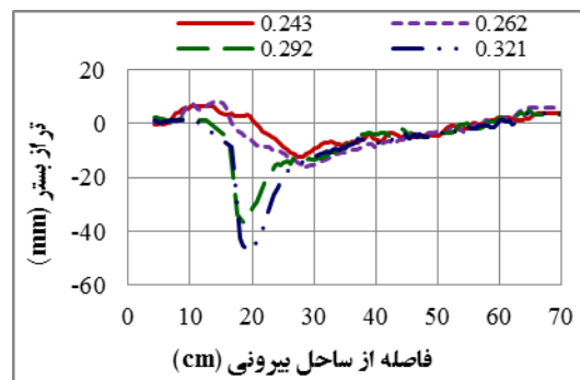
شکل ۵- پروفیل‌های عرضی مقاطع حداکثر عمق آبستگي در پنجه سازه به ازای اعداد فرود مختلف برای ترکیب سرریز و تیغه افقی
