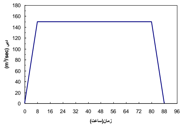
شکل ۳- الف-هیدروگراف ورودی، ب- رابطه دبی- اشل مقطع خروجی
