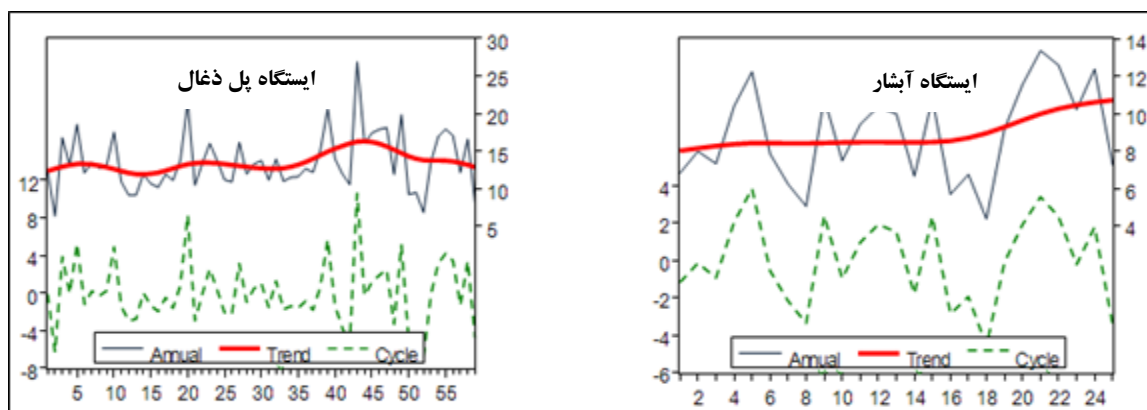
شکل ۷- روند تغییرات دبی با مدل هودریک- پریسکات در ایستگاه های هیدرومتری آبشار و پل ذغال در حوضه مجاور سردآبرود
