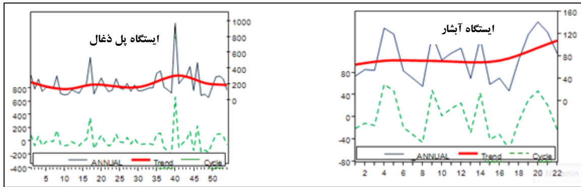
شکل ۹ - روند تغییرات رسوب با مدل هودریک- پریسکات در ایستگاه های هیدرومتری آبشار و پل ذغال در حوضه مجاور سردآبرود
