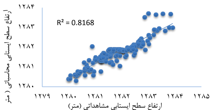
شکل ۱۰- نمودار ارتفاع سطح ایستابی مشاهده‌ای و محاسبه‌ای با استفاده از معادله دیفرانسیلی
