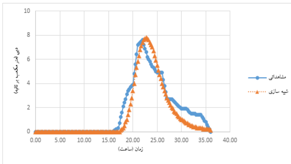
شکل ۴- هیدروگراف مشاهده‌ای و شبیه‌سازی شده واقعه‌ی ۱۳۸۸/۱۰/۱۰ بعد از واسنجی مدل HEC-HMS
