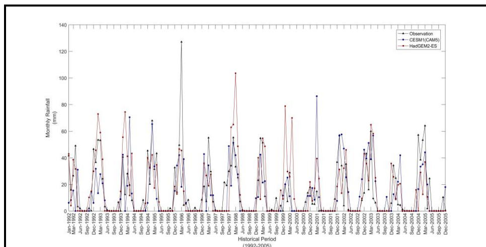
Fig. 2- Time series of the simulated and observation monthly precipitation شکل ۲- مقایسه بارندگی ماهانه مشاهداتی و شبیه‌سازی توسط دو مدل برتر
