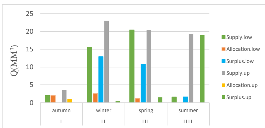
شکل ۷- مقایسه شاخص عرضه نسبی آب آبیاری در چهار فصل تحت سناریو کم
